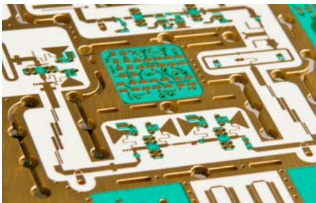
Hochfrequenz Leiterplatte mit Rogers Material
